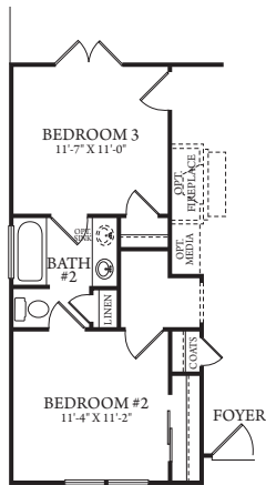
OPT. BEDROOM 3
