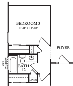
OPT. BEDROOM 3
