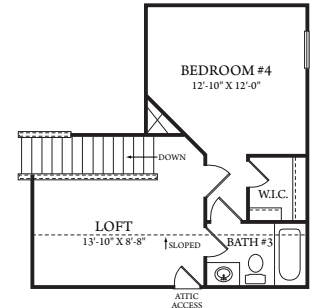
OPT. BEDROOM 4/ LOFT
